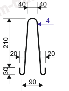
Монтажная петля
